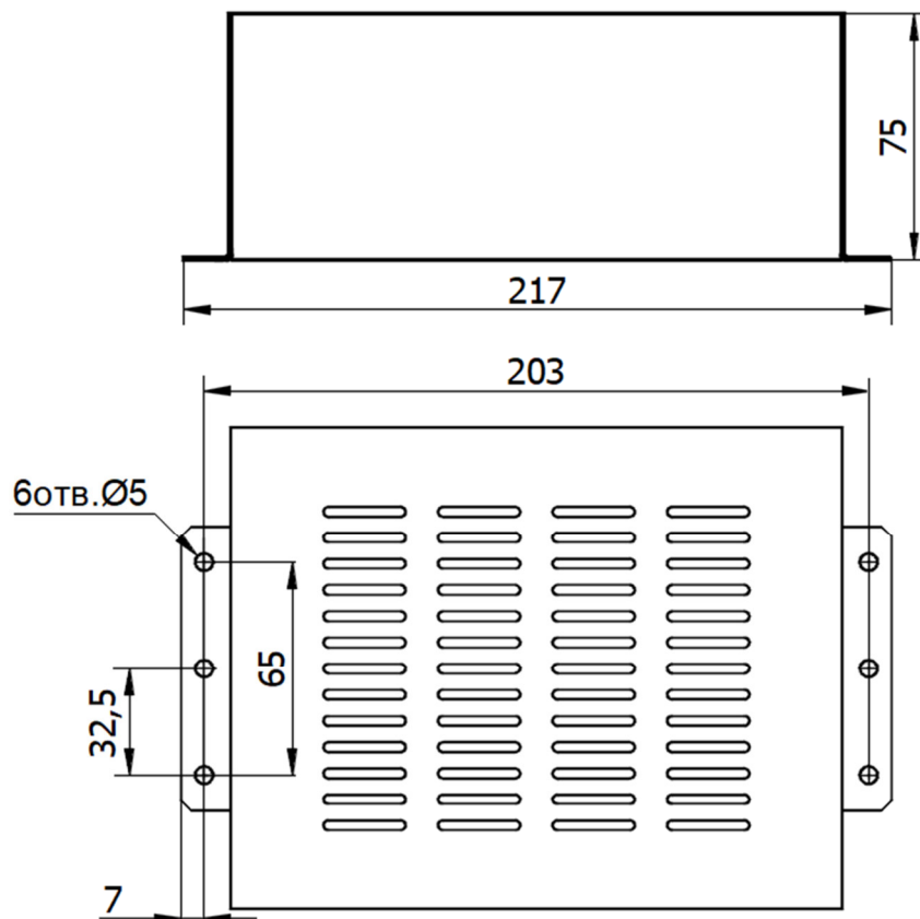
Рисунок 1 - Габаритные размеры защитного кожуха
